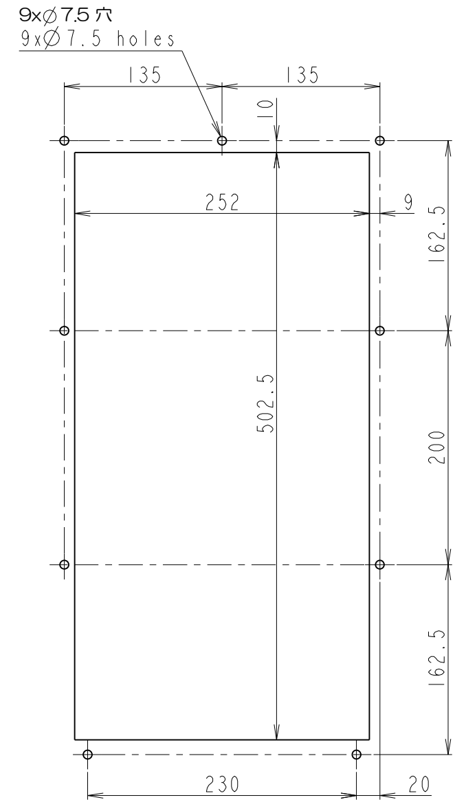
パネルカット寸法 Panel cutout dimension
